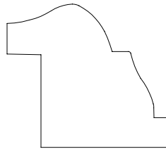
BACKBAND 61062 1 1/16" X 1 11/64"
